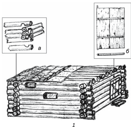
Рис. 5. Однокамерные срубные постройки с плоской крышей. 1 – однокамерная срубная постройка с плоской крышей на поселении Линёво-1: а – способ угловой вязки бревен, б – устройство входной двери (реконструкция авторов); 2 – однокамерное жилище-зимник с плоской крышей на плато Укок, Алтай, фото В.П. Мыльникова, 1991 г.
