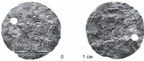
Рис. 2. Венгерская монета с Таманского городища (по: [Гончаров, Чхаидзе, 2007]).
