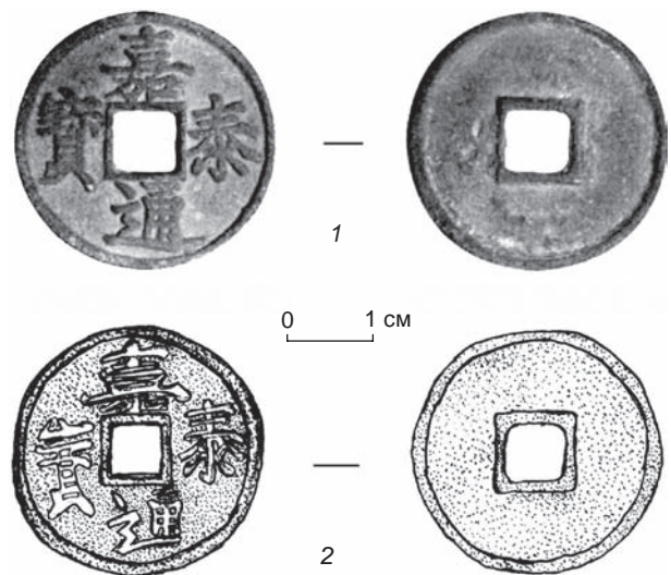
Рис. 4. Китайские монеты с Северного Кавказа. 1 – г. Маджар (по: [Обухов, 2001, с. 129, рис. 1]), 2 – Северо-Западный Прикаспий (прорисовка М.П. Севостьянова).
