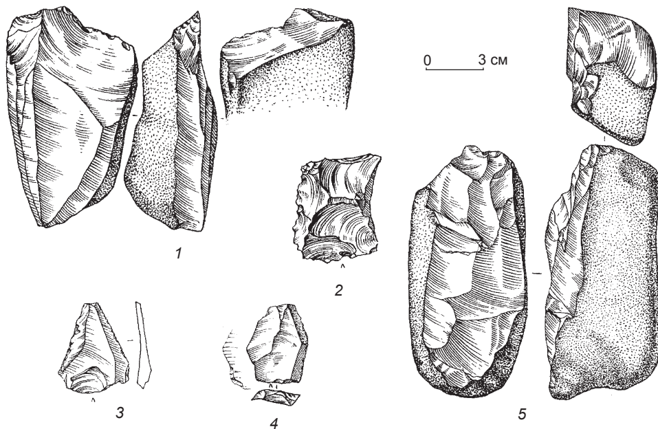
Рис. 20. Каменный инвентарь из слоя 7 пещеры Окладникова (по: [Деревянко, 2009б]). 1, 5 – нуклеусы; 2 – скребло; 3, 4 – острия леваллуа.
