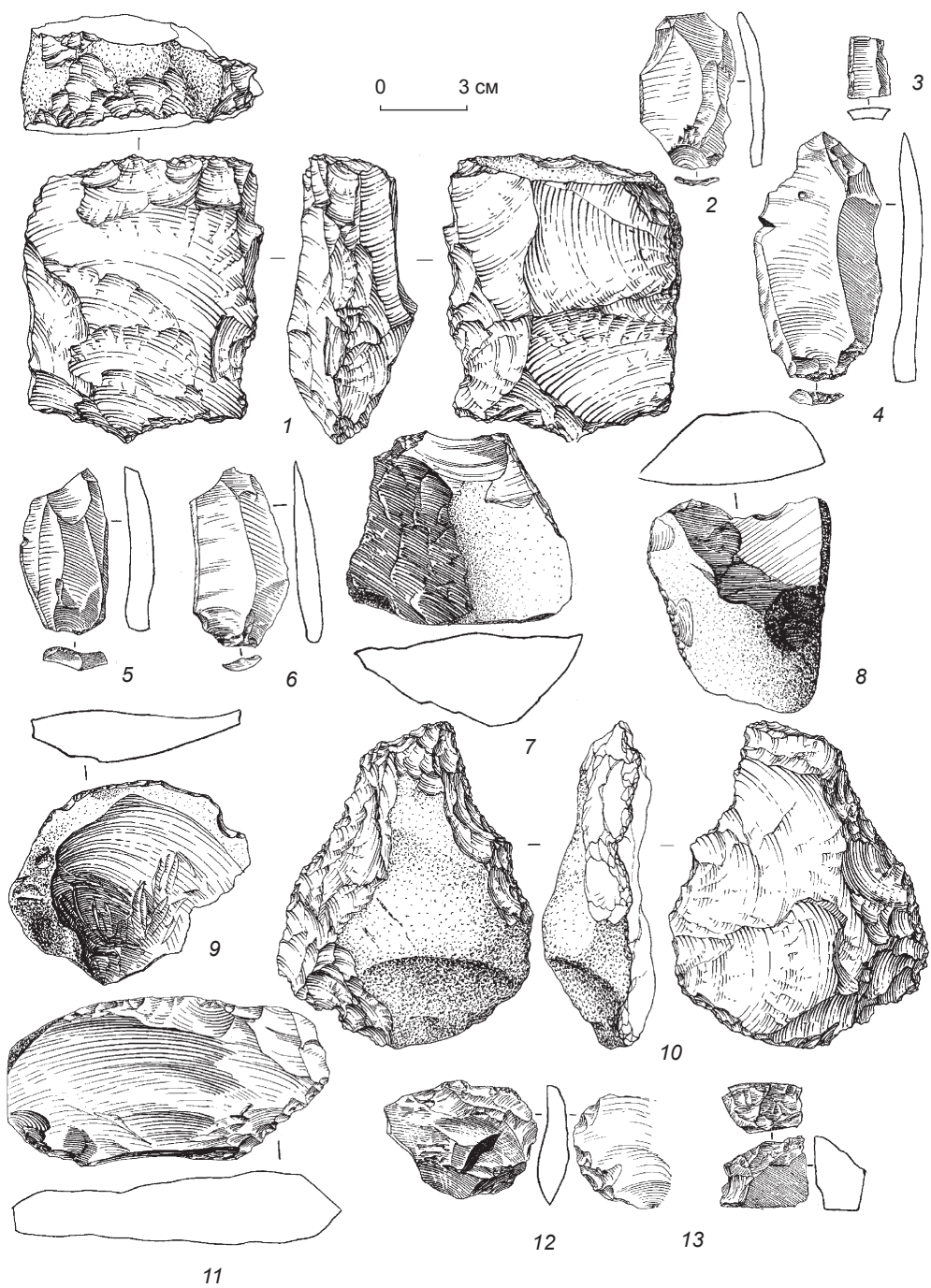
Рис. 29. Каменный инвентарь из горизонта 3 раскопов 1, 2 местонахождения Орхон-1 (по: [Дервянко, 2009б]).
