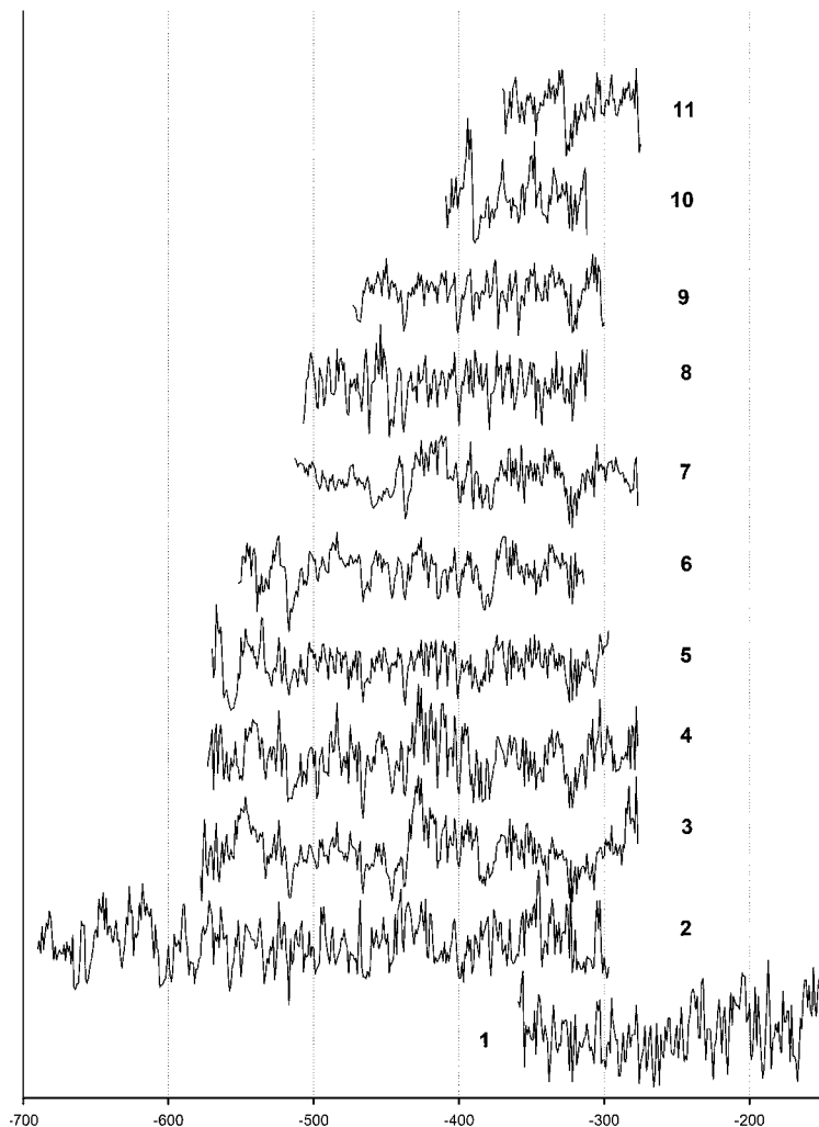
Рис. 2. Перекрестное датирование дендрохронологических шкал курганов Алтая и Монголии и длительной древесно-кольцевой шкалы «Монгун-Тайга» с установлением календарных дат археологических памятников.
