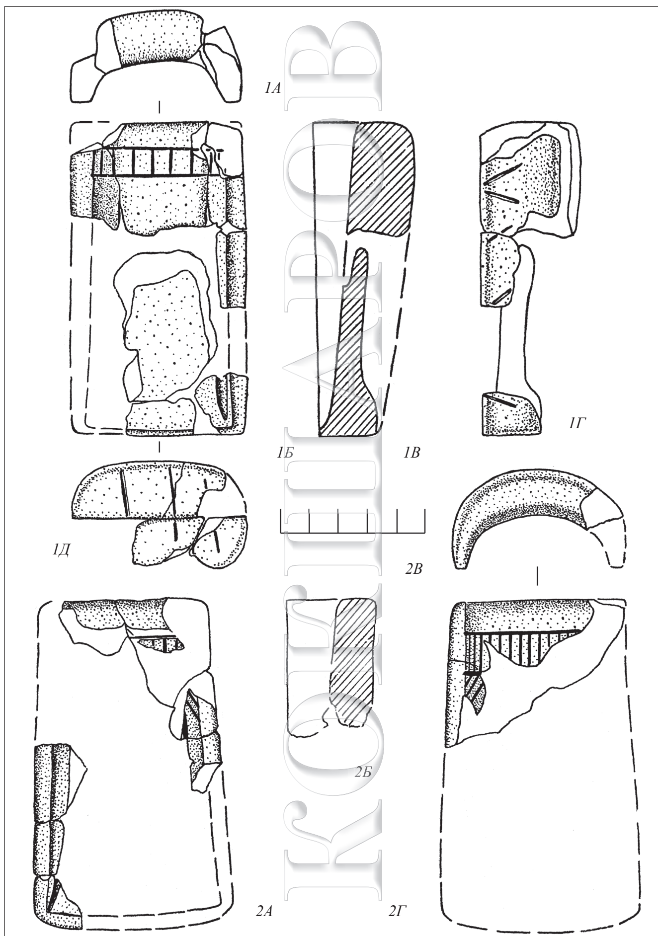
Рис. 232. Могильник Сатыга XVI. Литейные формы кельтов из могилы 5
