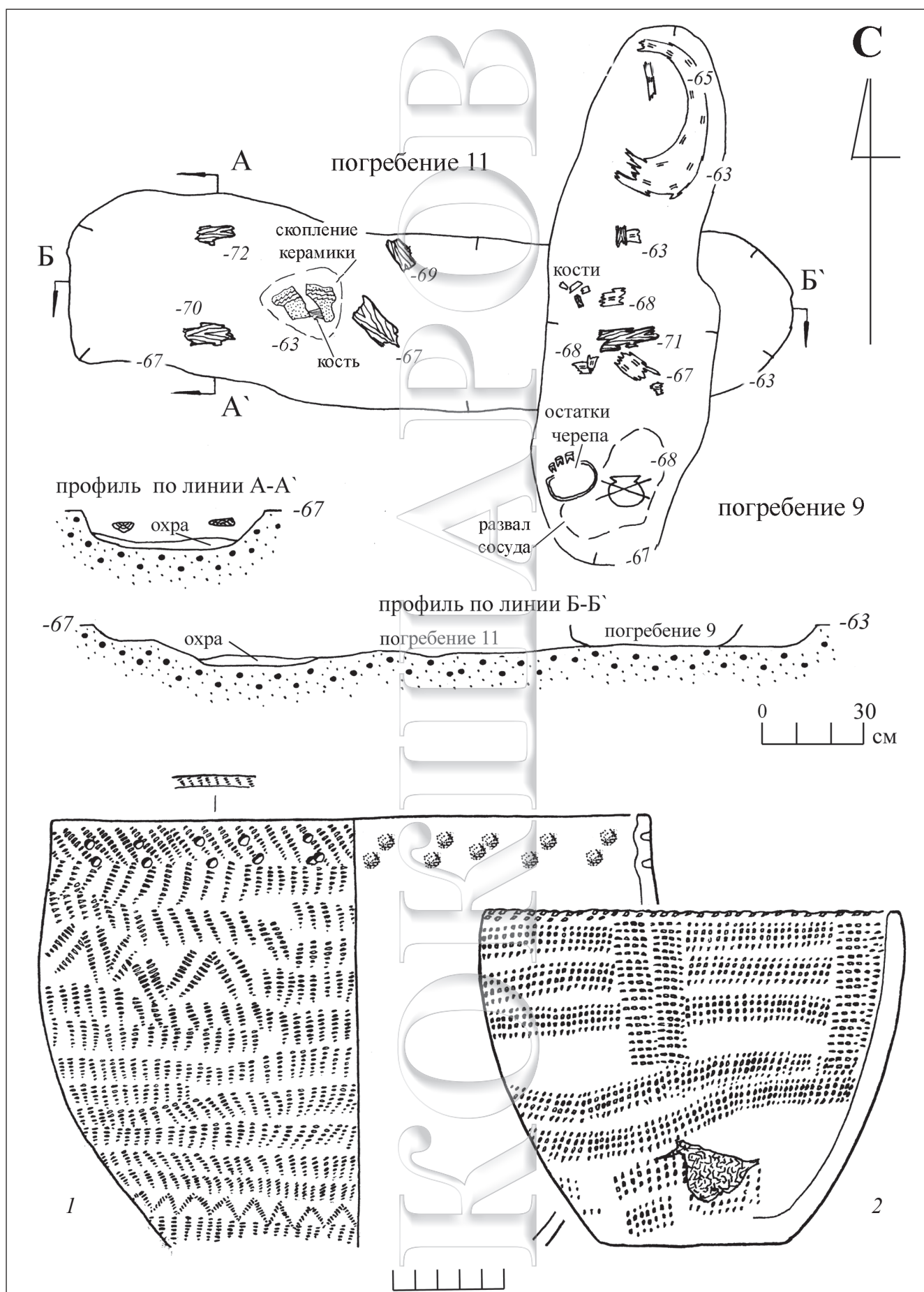
Рис. 242. Могильник Сатыга XVI. Планы и профили погребений 9 и 11 (по Е. М. Беспрозванному [1988, рис. 12]): 1 – горшок из погребения 9; 2 – сосуд из погребения 11
